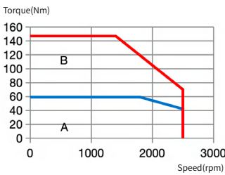
IMS20A-20M25D18C-4-***
