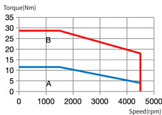
IMS20B-13H18C15C-**-***
