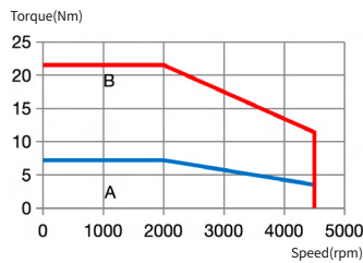
IMS20B-13H85B15C-**-***
