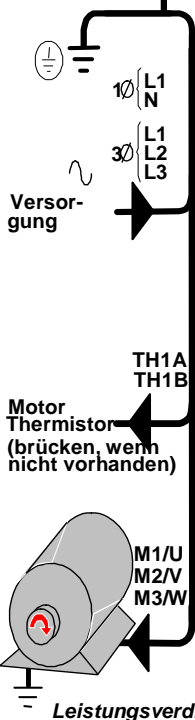
Leistungsverdrahtung
