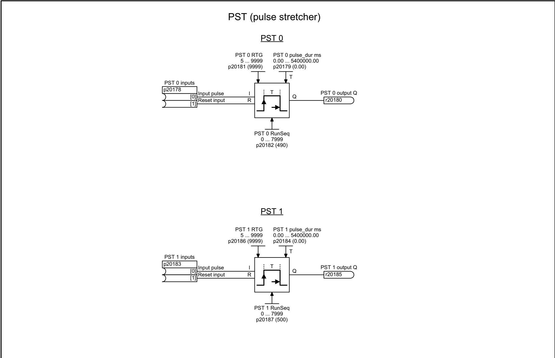
Fig. 3-133 7234 – PST 0 ... 1
