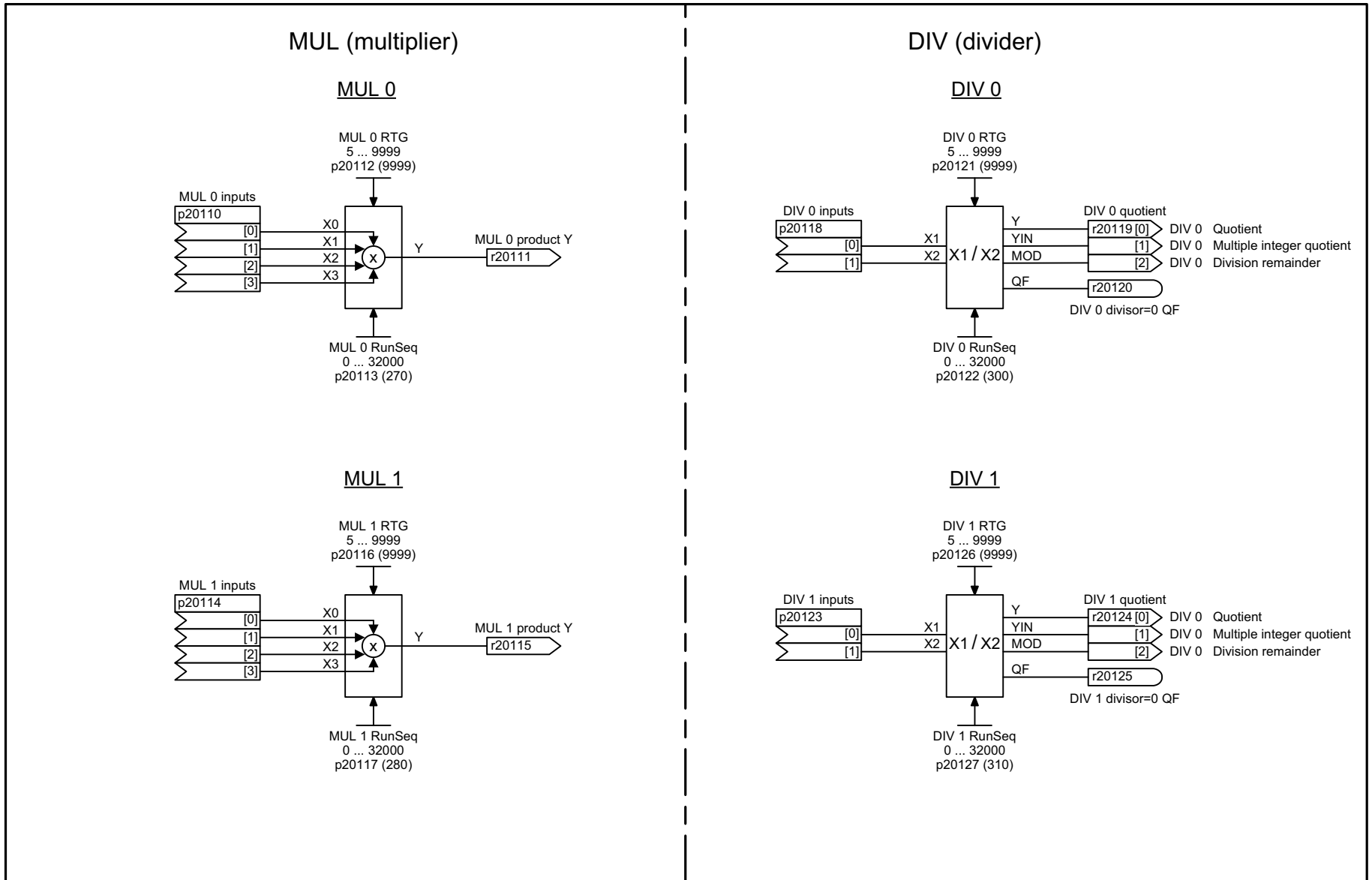
Fig. 3-126 7222 – MUL 0 ... 1, DIV 0 ... 1
