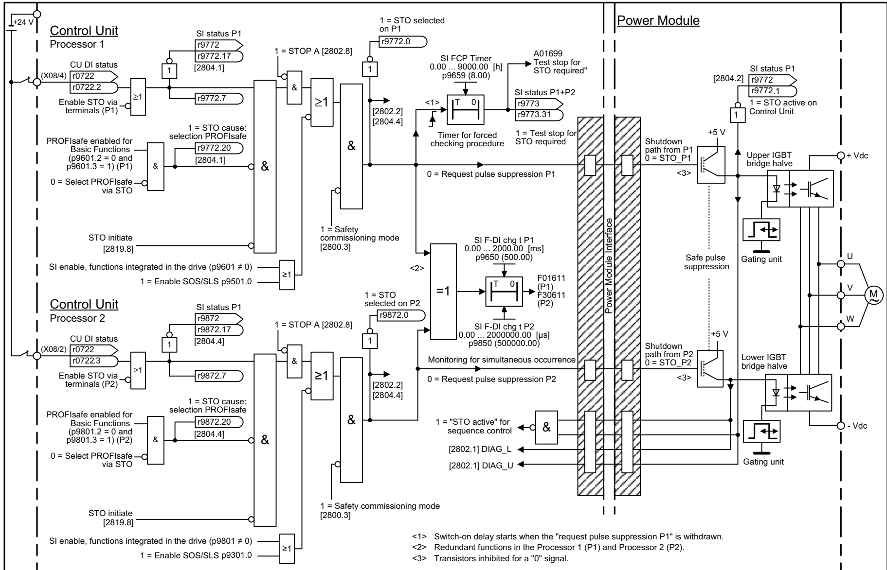
Fig. 3-62 2810 - STO (Safe Torque Off)
