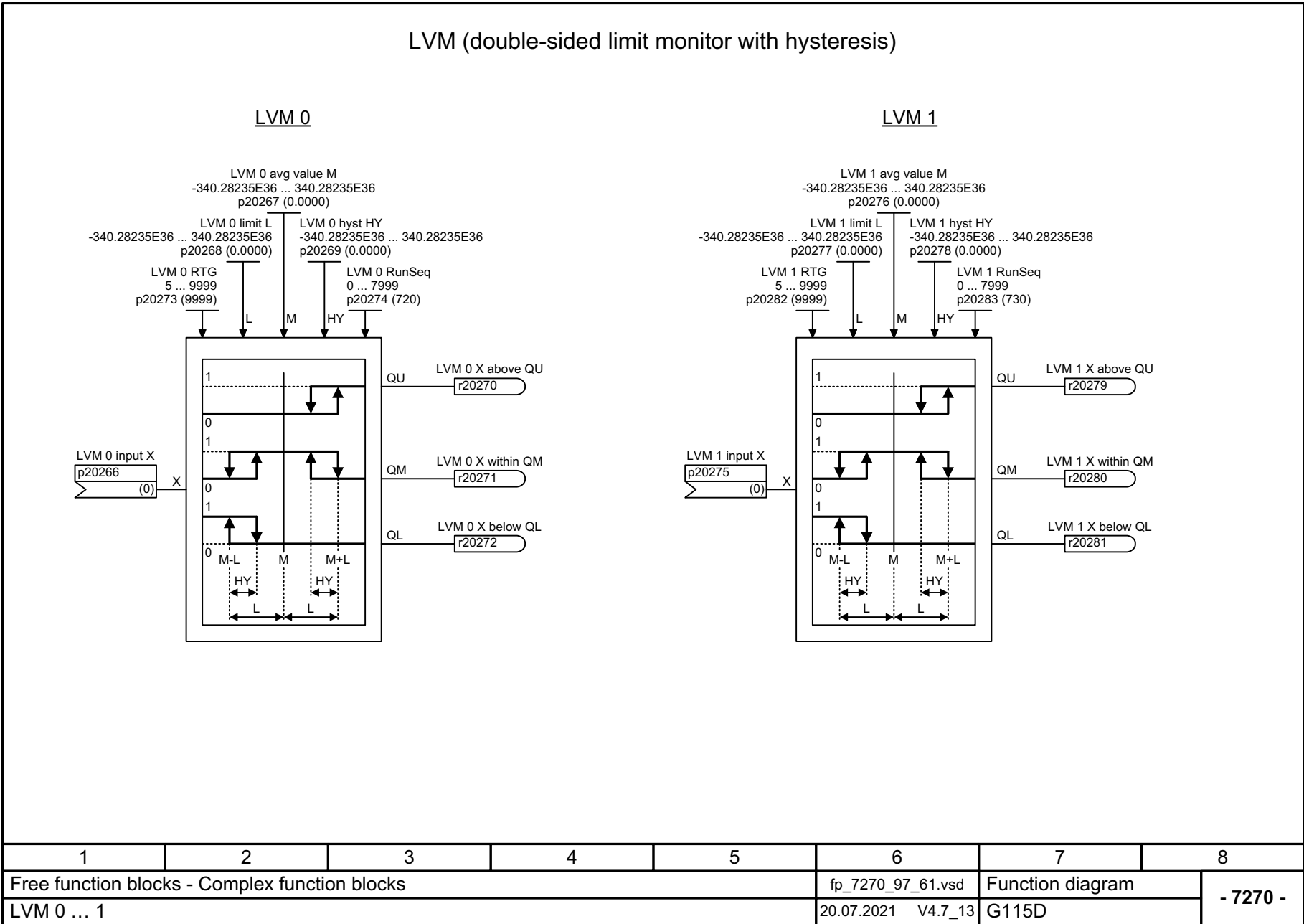
Fig. 3-139 7270 - LVM 0 ... 1
