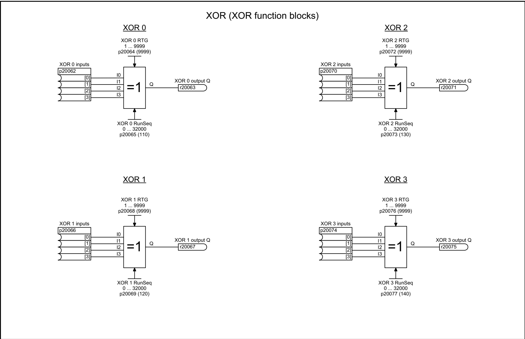
Fig. 3-123 7214 – XOR 0 ... 3
