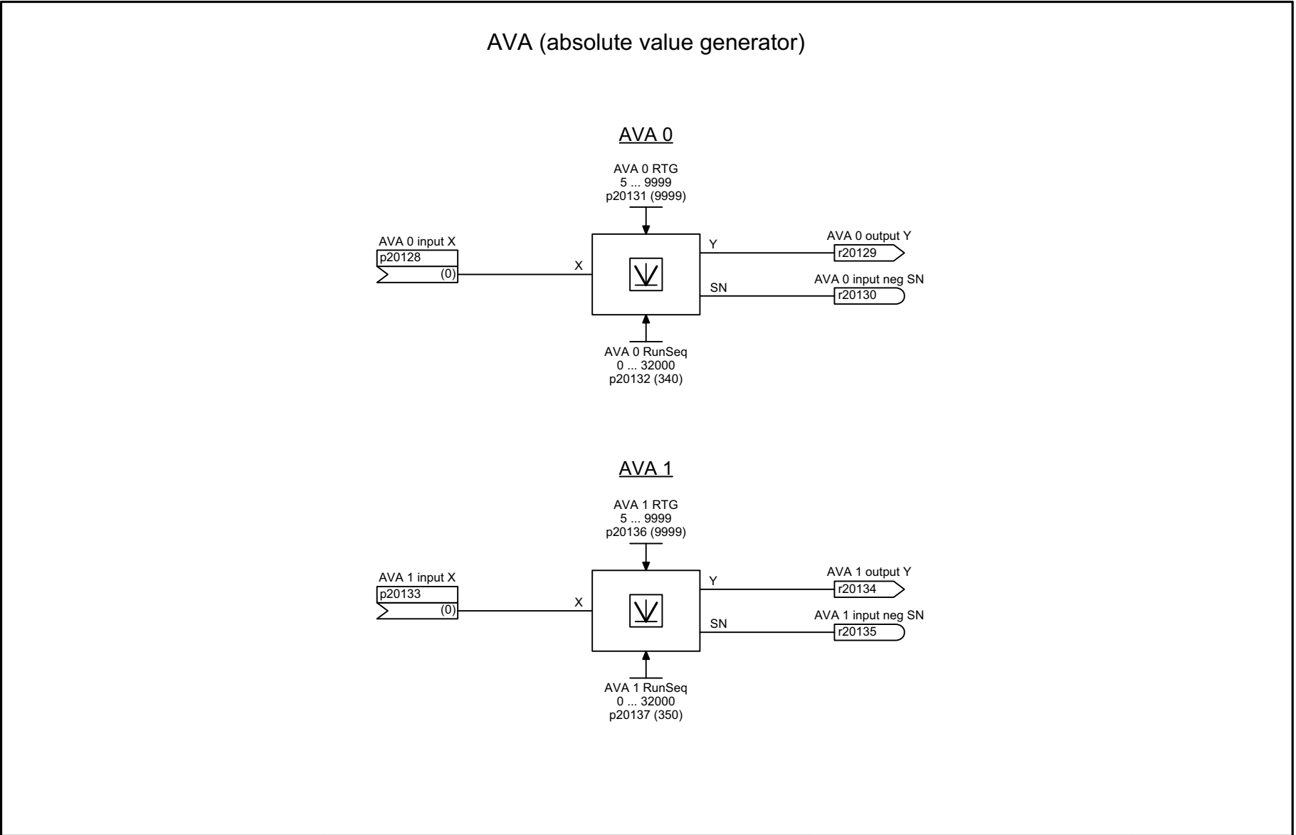
Fig. 3-127 7224 – AVA 0 ... 1
