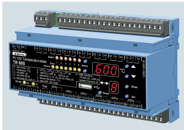
L94 Pt100 Ziehl TR600
