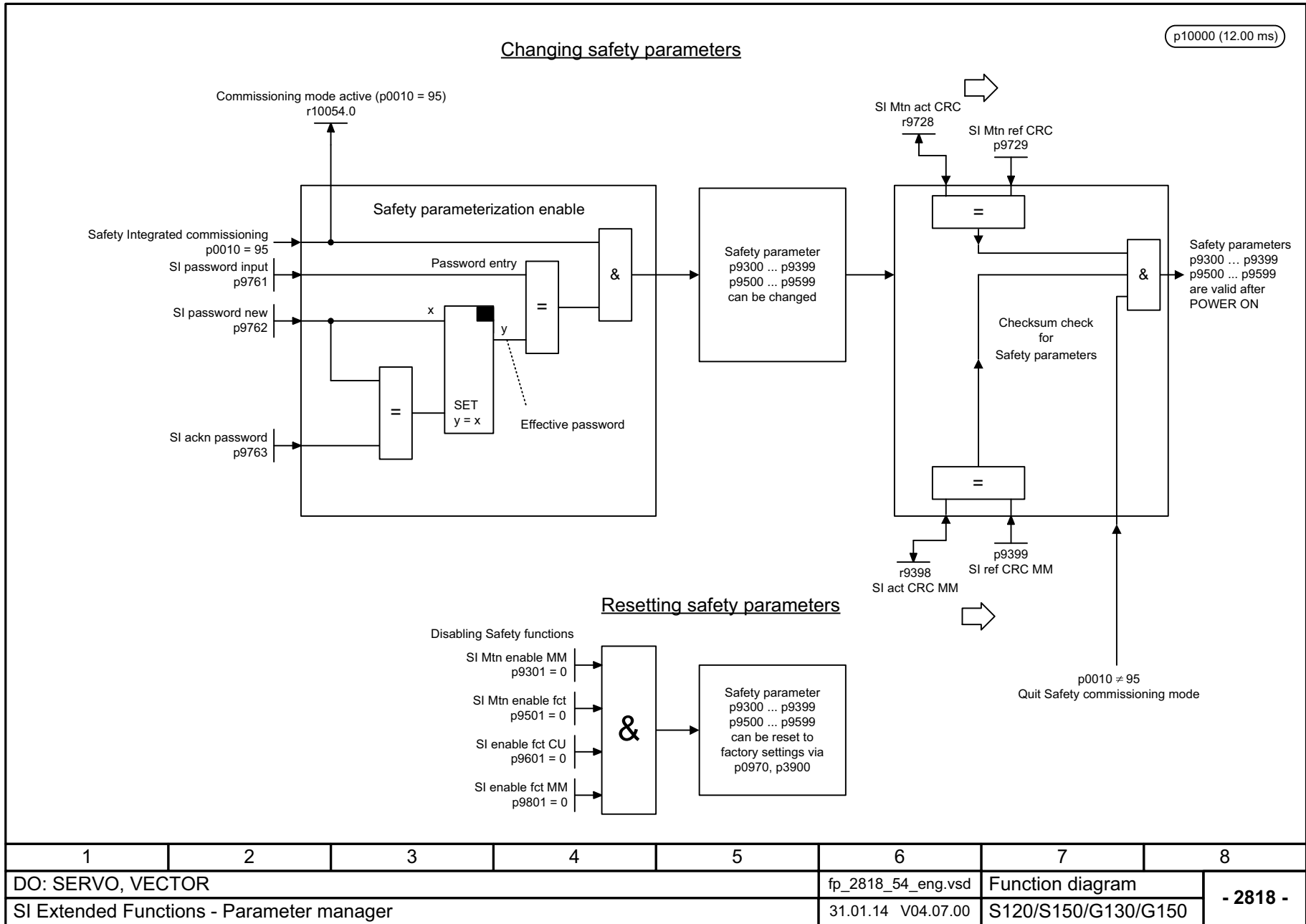
Fig. 3-116 2818 – Parameter manager
