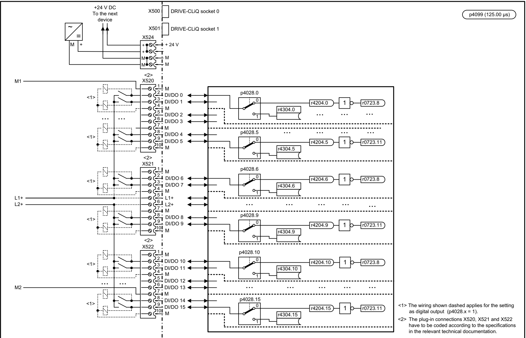
Fig. 3-346 9419 – Overview
