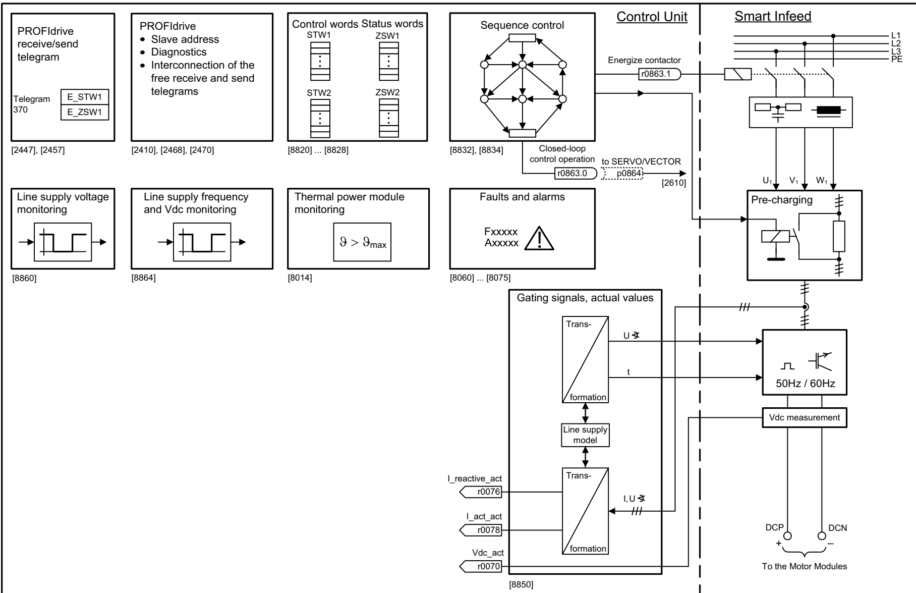
Fig. 3-307 8810 – Overview
