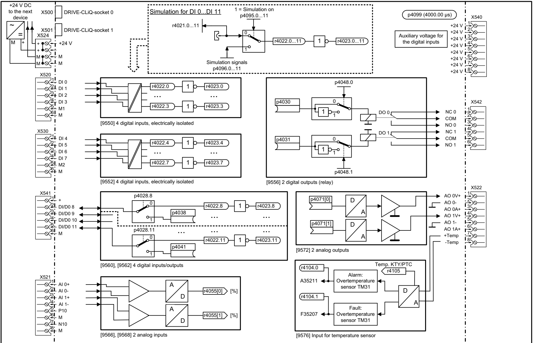
Fig. 3-347 9549 – Overview
