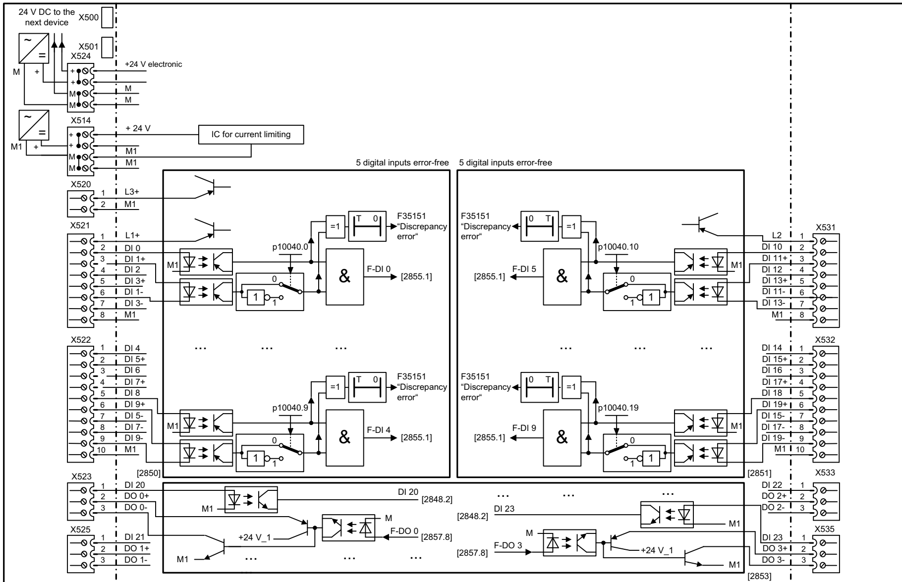
Fig. 3-128 2846 – TM54F overview
